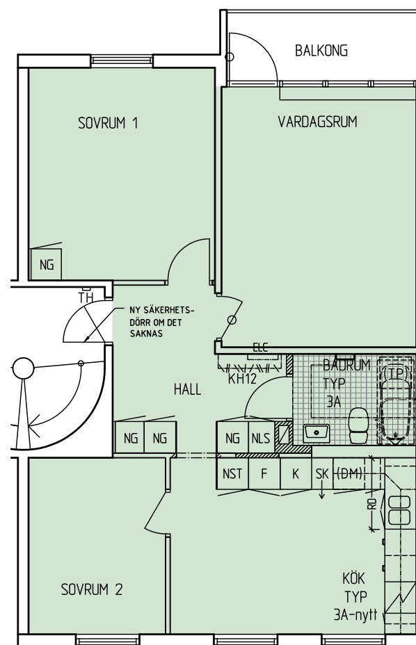
NYTT UTFÖRANDE
