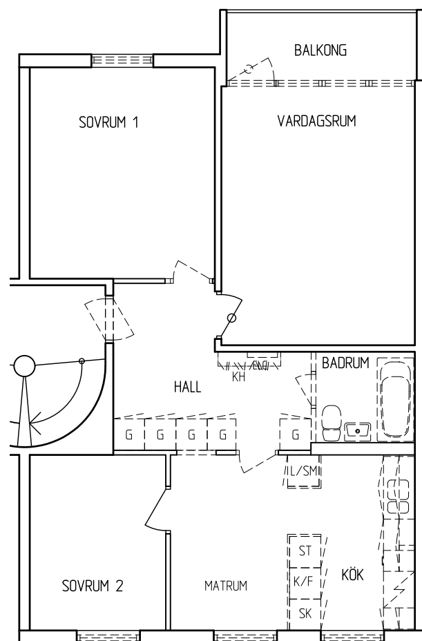
BEFINTLIGT UTFÖRANDE
